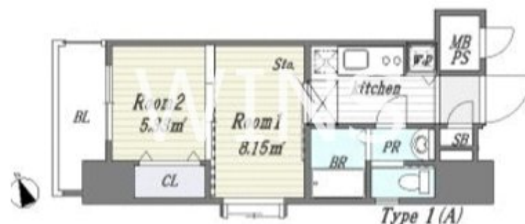
【間取り図】
