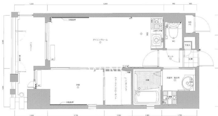
【間取り図】
