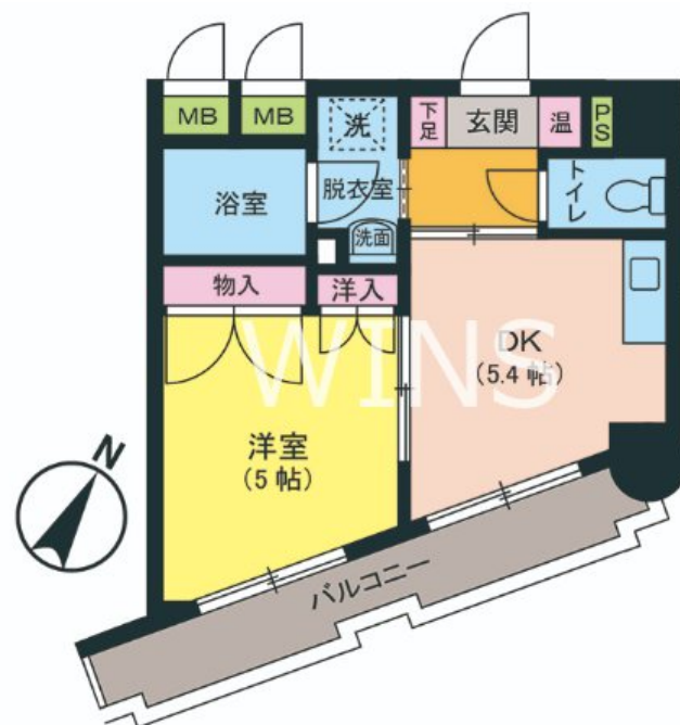
【間取り図】
